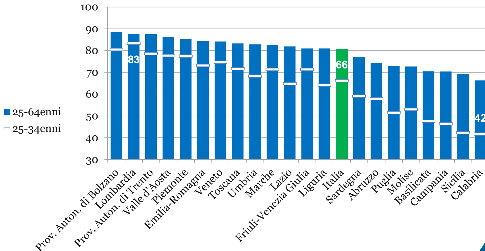
Tassi di occupazione degli adulti laureati in Italia, per classe di età (2017)
