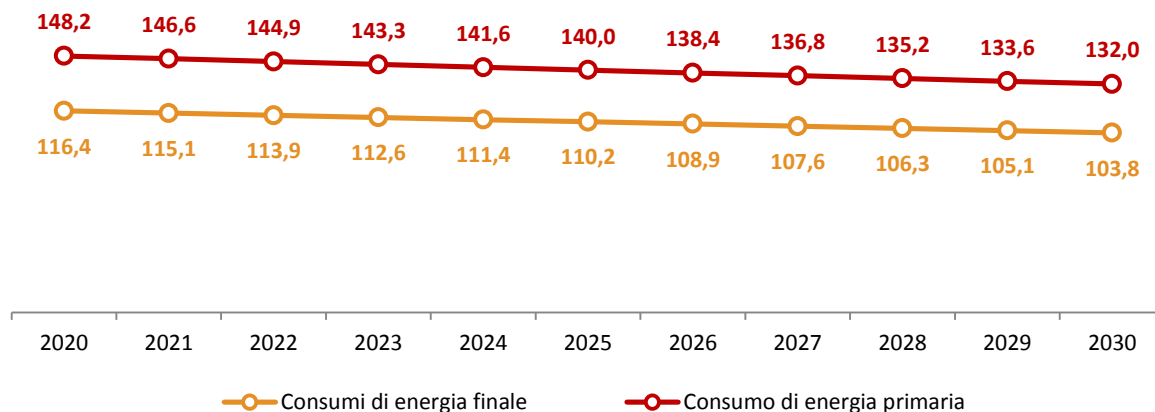
Figura 17 - Traiettorie dei consumi di energia primaria e finale (Mtep) nel periodo 2020-2030 [Fonte: RSE]
